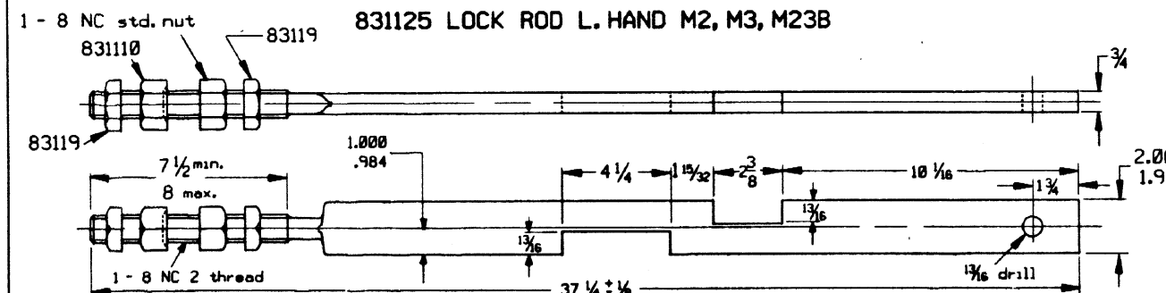
831123 LOCK ROD R, HAND M2, M3, M23B
