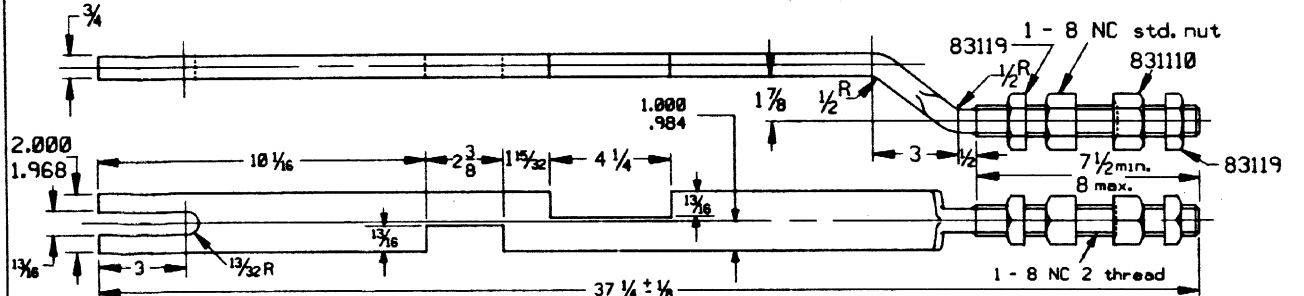
831125 LOCK ROD L. HAND M2, M3, M23B
