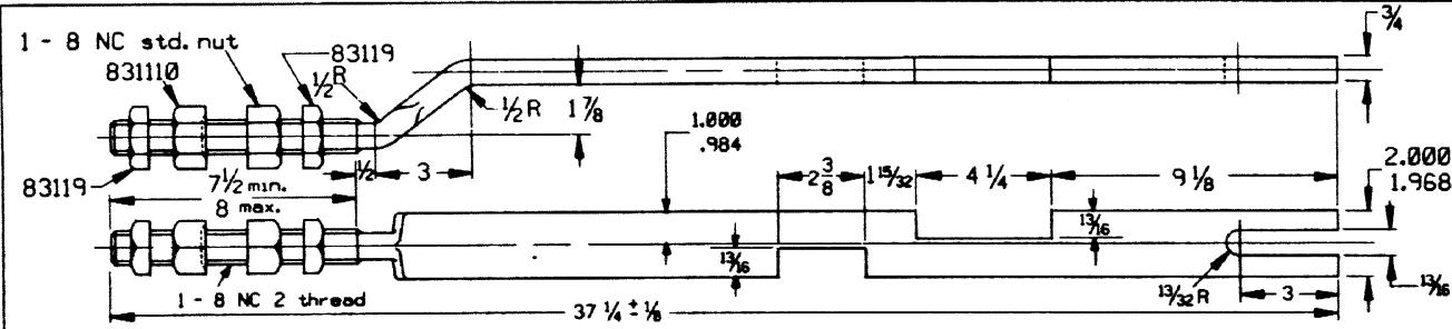
831124 LOCK ROD R. HAND M2, M3, M23B
